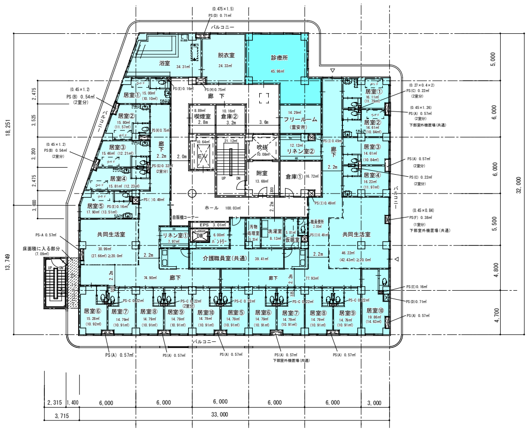
ショートステイ①(個室型) 3階平面図 1:200 特養③(個室型)
