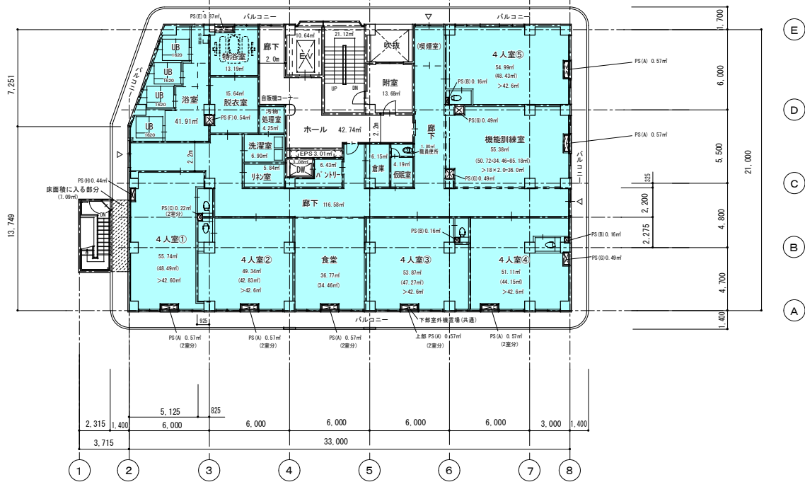
特装⑤ (多床室型) 6階平面図 1:200 特装⑥ (多床室型) (4人室有効面積 42.60㎡以上必要)
