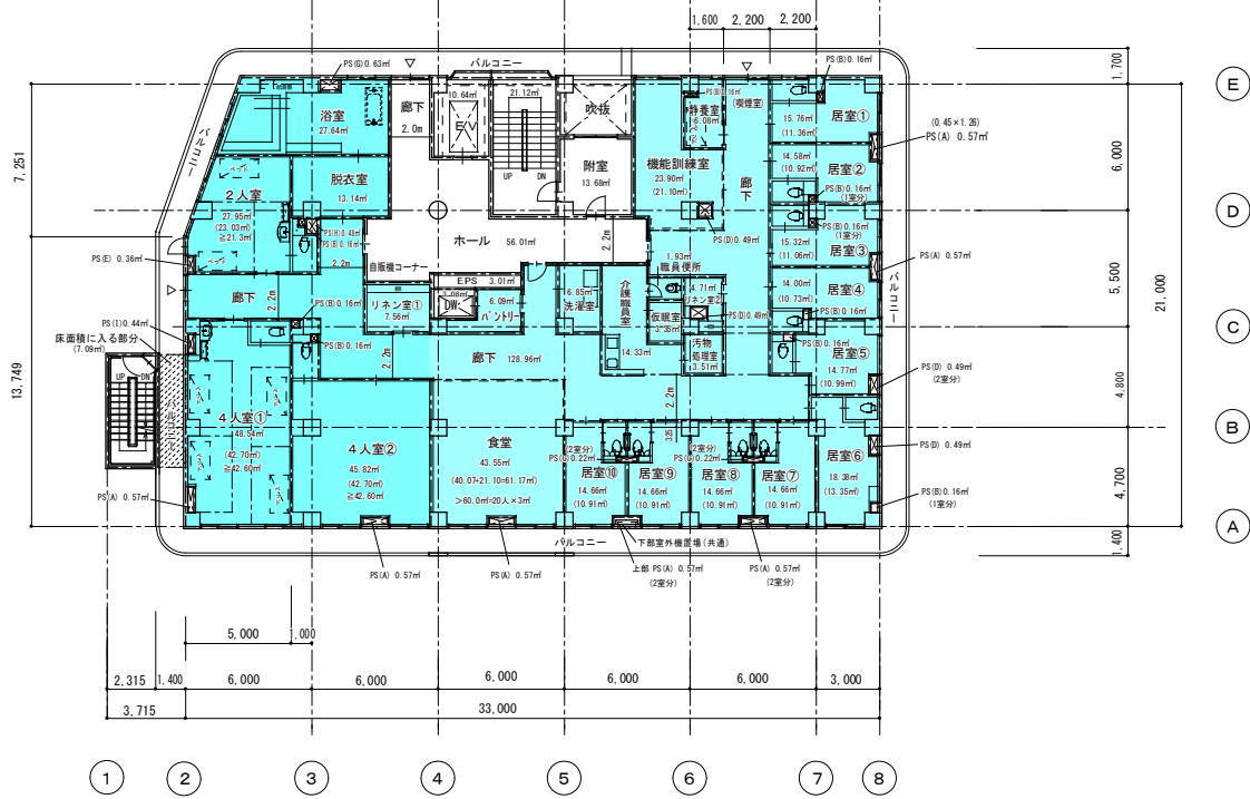
特装⑥ (多床室型) 5階平面図 1:200 ショートステイ②(個室型)
